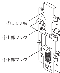
図 1 AT-DRMT-J01 外觀 (本体と DIN レール取り付け金具を取り外した状態)
