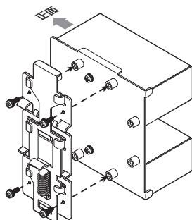
図7 DIN レール取り付け金具の固定
