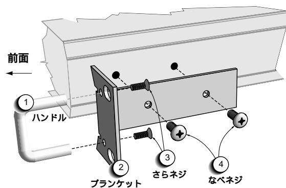
図 1: ハンドルおよびブラケットの取付け方
