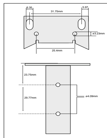
図 2: RKMT-5 の外形寸法
