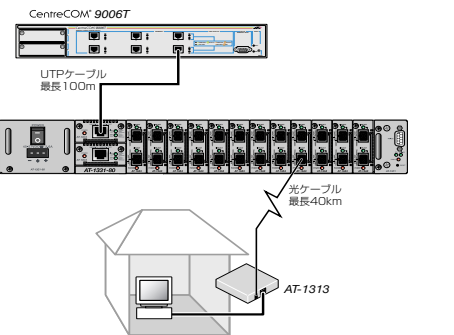
図5 接続例
