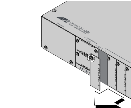
図2 カバーパネルの取り外し
