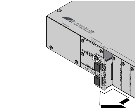
図3 ラインカードの取り外し
