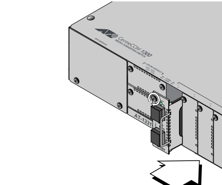
図4 本製品の取り付け
