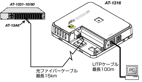
図9 接続例
