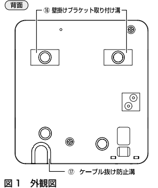
図1 外観図
