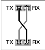
図7 ケーブル接続図
