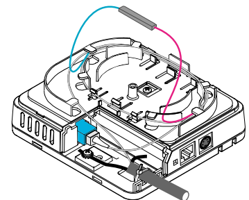
図6 光コードのスプライシング
