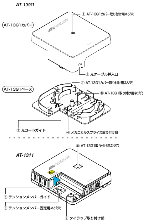
図1 外観図
