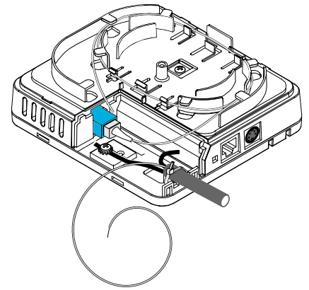
図5 光コードの巻き付け
