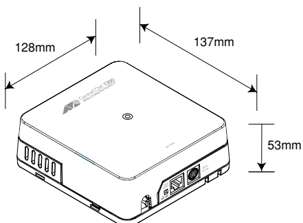
図8 製品寸法図
