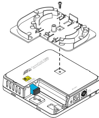
図2 本体の固定
