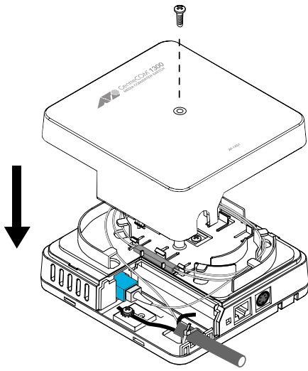
図7 カバーの取り付け
