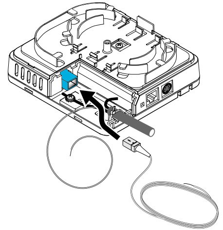
図4 光コードの接続
