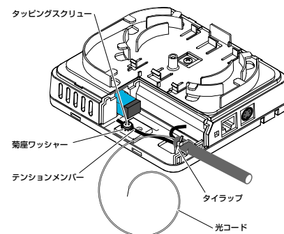
図3 光ケーブルの固定
