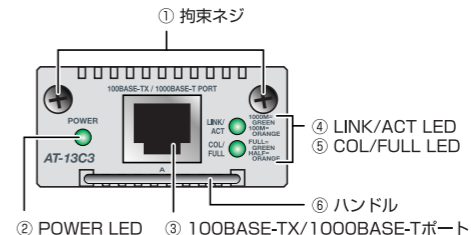
図 1 AT-13C3 前面図
