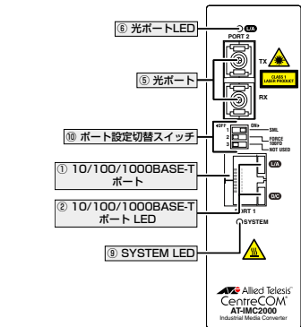
図 1 AT-IMC2000T/SC 前面
