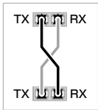
図 10 光ファイバーケーブルの接続
