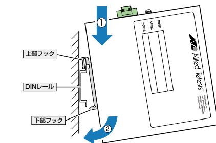
図 9 DIN レールへの取り付け
