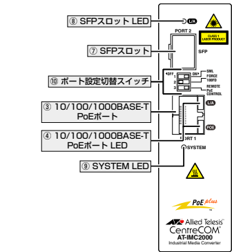
図 3 AT-IMC2000TP/SP 前面
