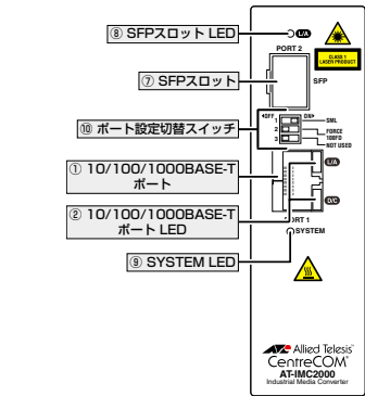
図 2 AT-IMC2000T/SP 前面
