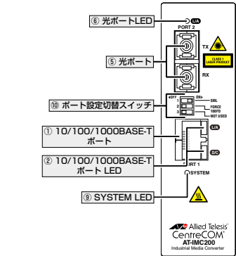
図 4 AT-IMC200T/SC 前面
