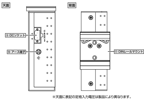
図 6 CentreCOM IMC シリーズ共通（天面・背面）
