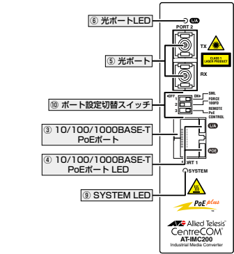
図 5 AT-IMC200TP/SC 前面
