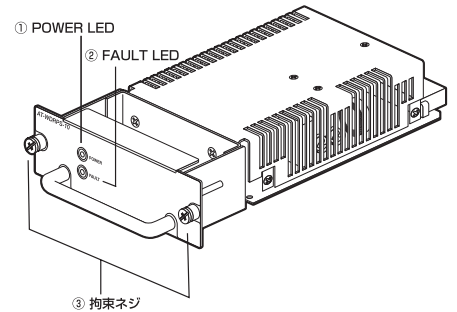
図 1 AT-WDRPS-10 外観図
