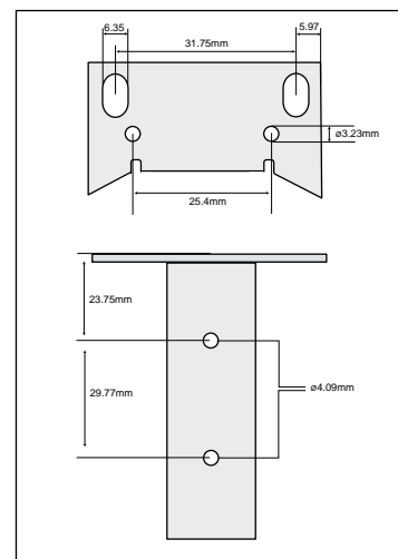
図2: C36C1 の外形寸法
