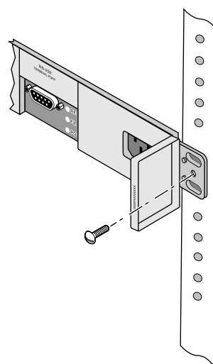
図 1.16 AT-CTSD4-1R1、AT-CTSD8-1R2 据置型シャーシのネジ止め
