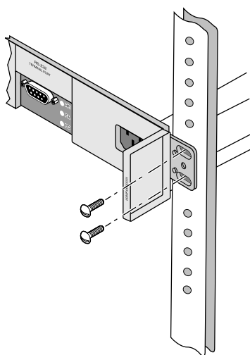
図 1.15 AT-CTSR4-1R1、AT-CTSR8-1R2 19 インチラック取付用のネジ止め
