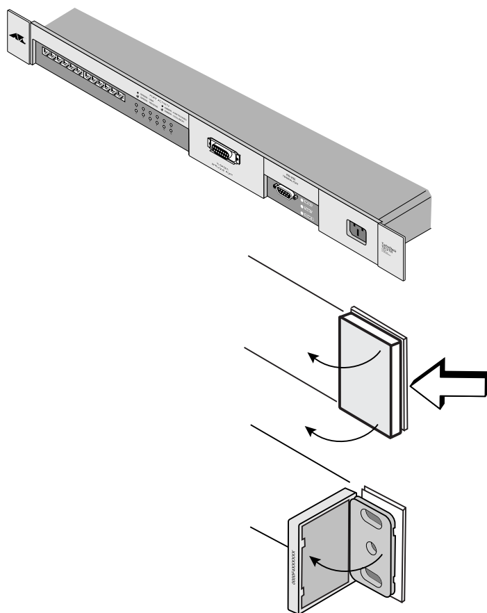
図 1.14 TS シリーズハブのブラケットカバーの開け方
