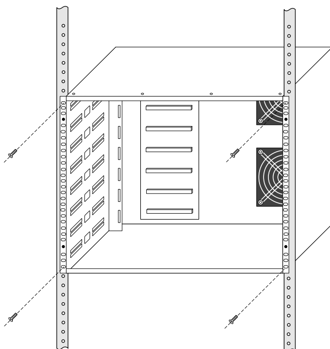
図 1.11 19 インチラックへの取り付け
