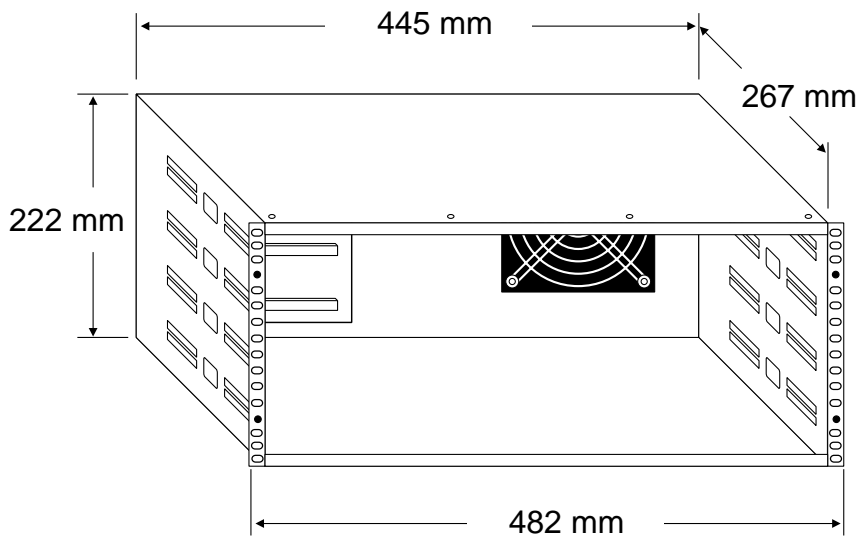
AT-CTSR4-1R1 外形寸法
