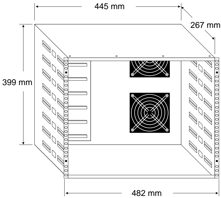
AT-CTSR8-1R1 外形寸法
