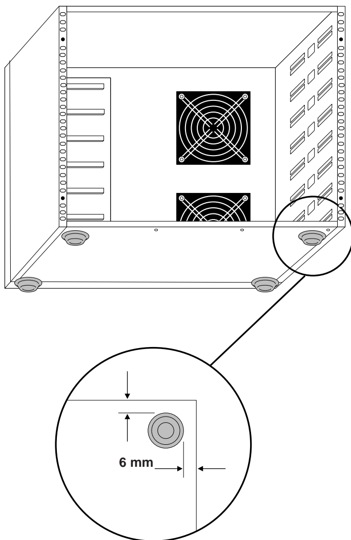
図 1.10 AT-CTSDS4-1R1、AT-CTSDS8-1R2（据置型シャーシ）のゴム足の取り付け
