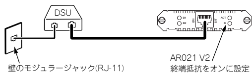
図A.6.4 DSUに直結の場合
