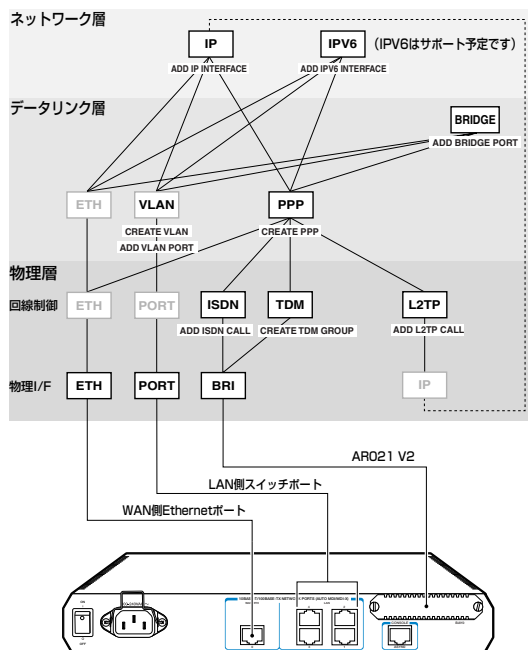
図 4.4.1 インターフェースの階層構造
