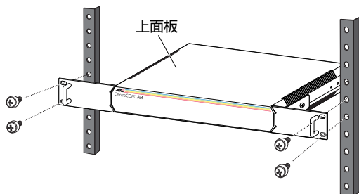
図2.2.3 ラックへの取り付け
