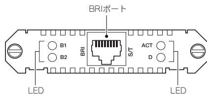
図 A.6.1 AR021 V2 背面パネル
