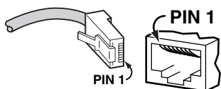
図 A.5.1 RJ-45 モジュージャック (左)、ジャック (右)
