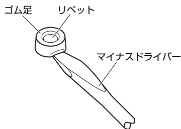
図 2.2.1 ゴム足の取り外し
