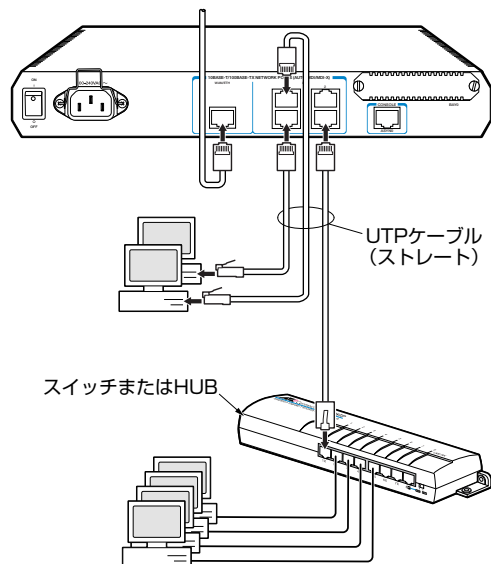
図 2.6.1 スイッチの接続
