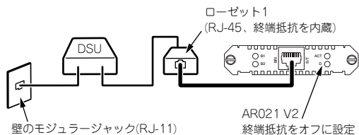
図A.6.3 ローゼット1つの場合
