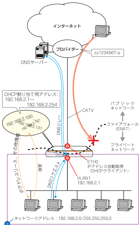
図 13.4.1 CATV による端末型の接続
