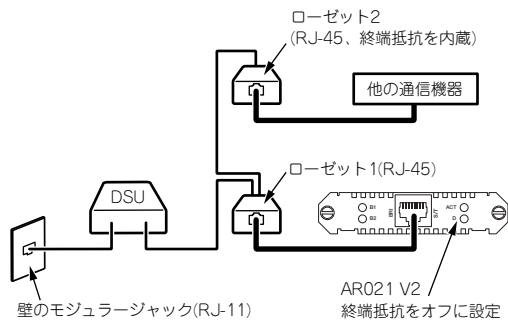
図A.6.5 ローゼット2つの場合
