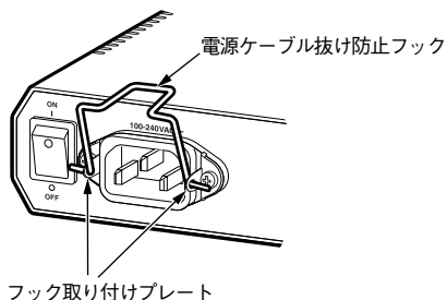
図 2.5.1 電源ケーブル抜け防止フックの取り付け
