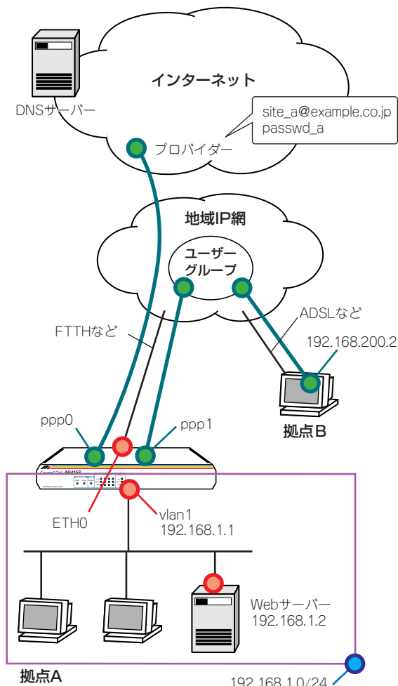
図13.7.1 インターネットとCUGサービスの同時接続(端末型)
