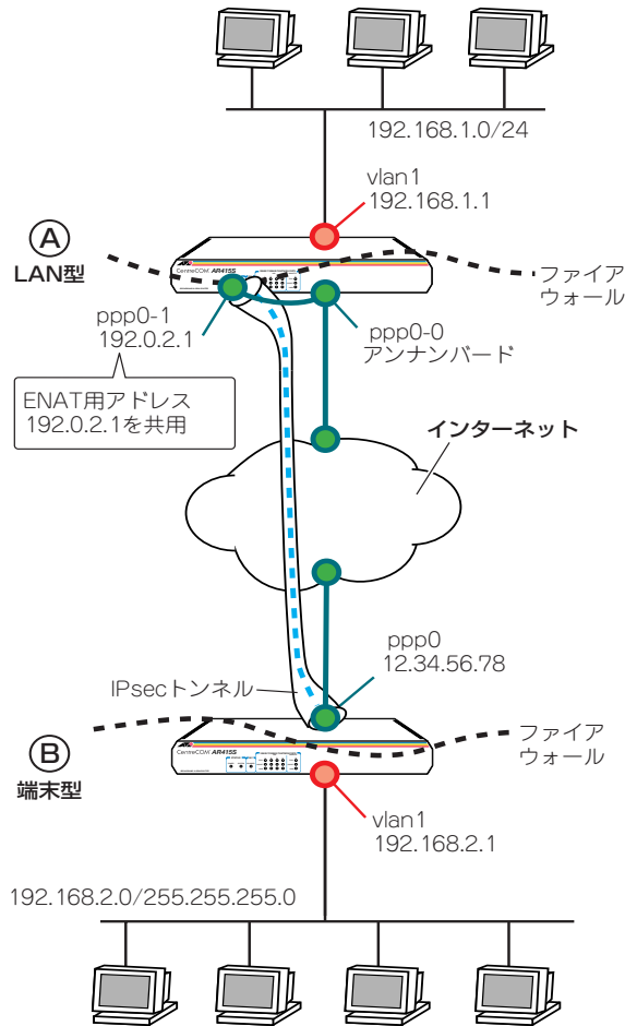
図 13.5.1 IPsec による接続
