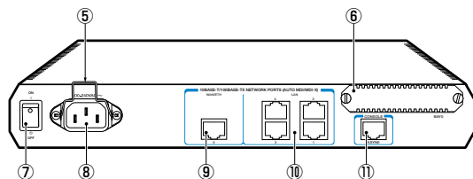
図 1.3.3 背面図
