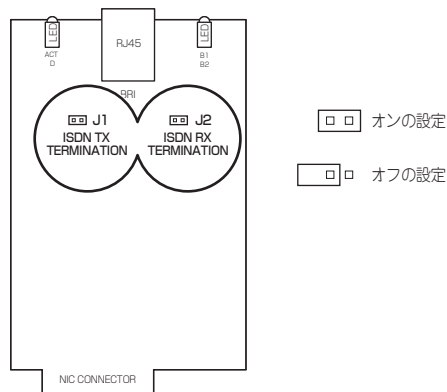
図 A.6.2 デフォルトのジャンパー設定
