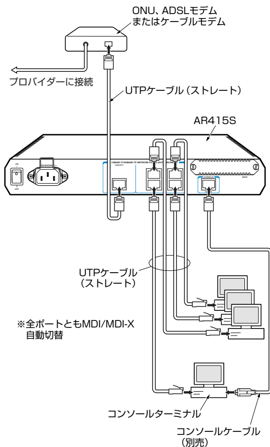
図 2.4.1 ブロードバンド系サービスを利用する場合の接続例
