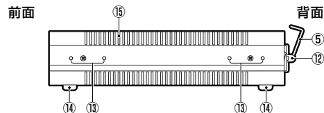
図 1.3.5 側面図
