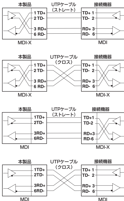
図 1.5.2 10BASE-T/100BASE-TX ケーブル結線図
