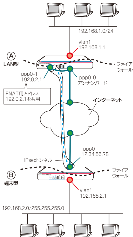
図 13.5.1 IPsec による接続
