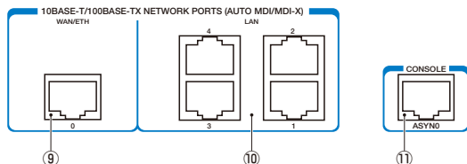
図 1.3.4 ポート
