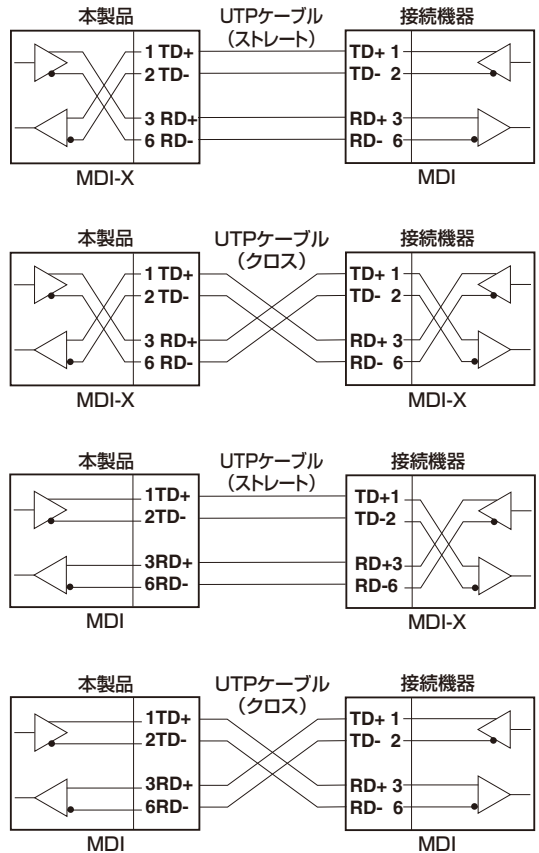
図 1.5.2 10BASE-T/100BASE-TX ケーブル結線図
