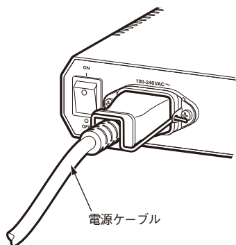
図 2.4.3 電源ケーブルのロック
