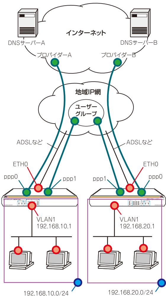
図 13.8.1 インターネットと CUG サービスの同時接続 (LAN 型)
