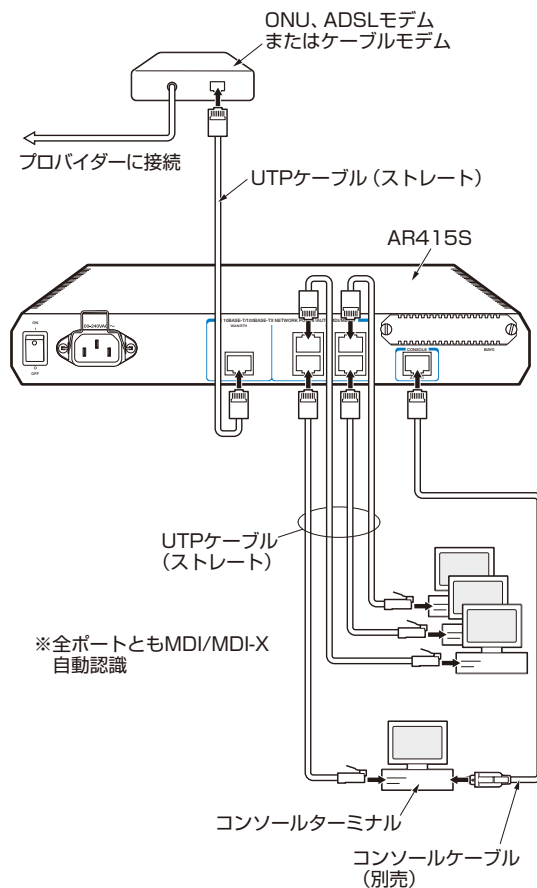
図 2.3.1 ブロードバンド系サービスを利用する場合の接続例
