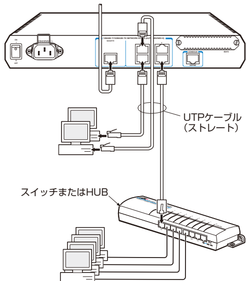
図 2.5.1 スイッチの接続
