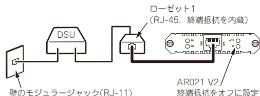
図 A.6.3 ローゼット1つの場合
