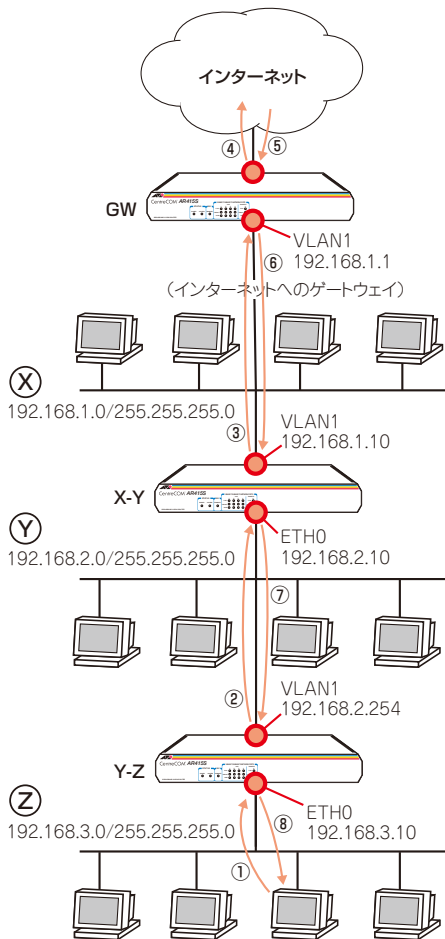
図 4.5.3 インターネットにも接続
