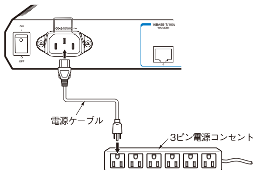
図 2.4.2 電源ケーブルの接続
