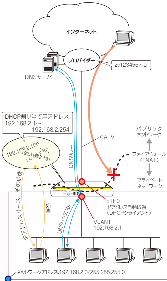
図 13.4.1 CATV による端末型の接続
