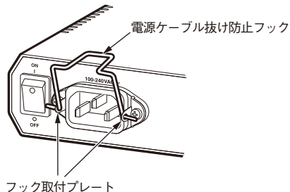
図 2.4.1 電源ケーブル抜け防止フックの取り付け
