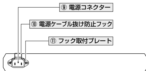
CentreCOM® 8316XL
