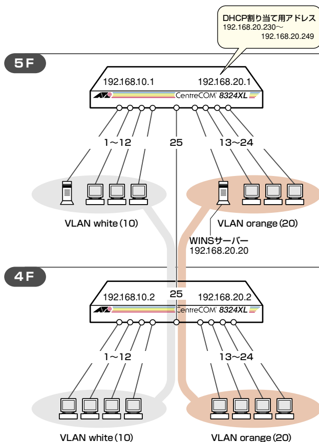
図 2 「タグ VLAN を使用した設定」構成例
