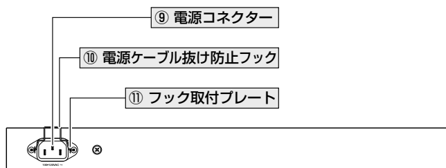
CentreCOM® 8316XL
