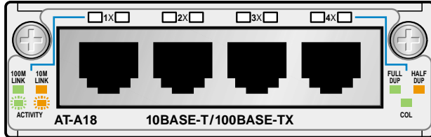
AT- A18 10BASE-T/100BASE-TX x 4ポート
