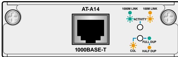
AT- A14 100BASE-TX/1000BASE-T x 1ポート
