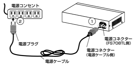
図8 電源ケーブルの接続
