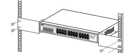
図 7 19 インチラックへの取り付け
