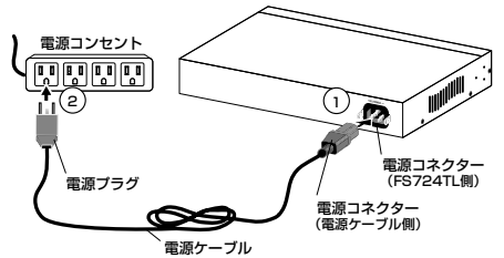
図 11 電源ケーブルの接続
