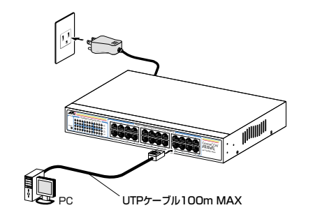
図 10 接続図
