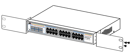
図 6 ブラケットの取り付け
