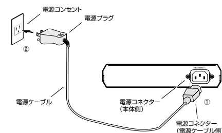
図5 電源ケーブルの接続 (図は AT-FS710/8)
