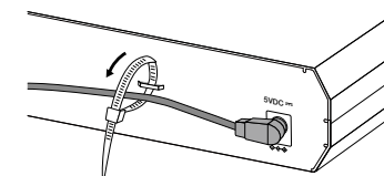
図7 DC 電源ケーブルの固定 (図は AT-FS710/8E)
