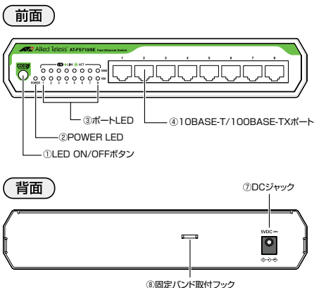
図 1 外観図
