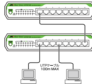
図8 カスケード接続 (図は AT-FS710/8)
