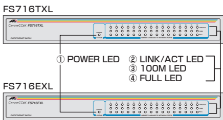
図 1 外観図 (前面)
