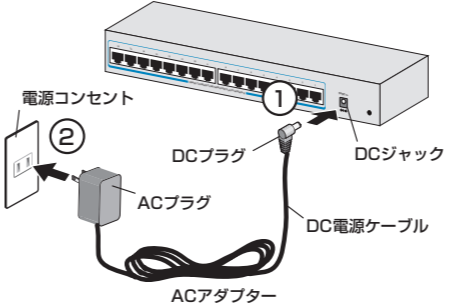
図7 ACアダプターの接続
