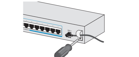
図8 DC電源ケーブルの固定
