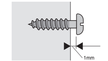
図4 タッピングスクリューのねじ込み
