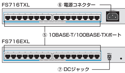
図 2 外観図 (背面)
