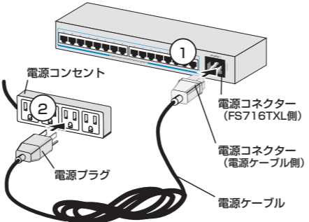
図6 電源ケーブルの接続
