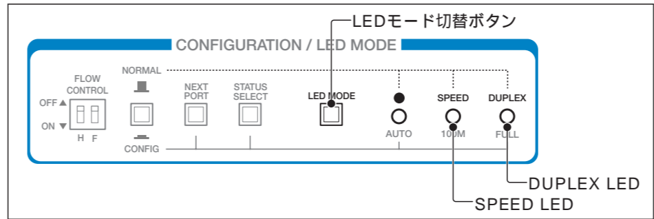
図3 LEDモード切替ボタン(拡大図)
