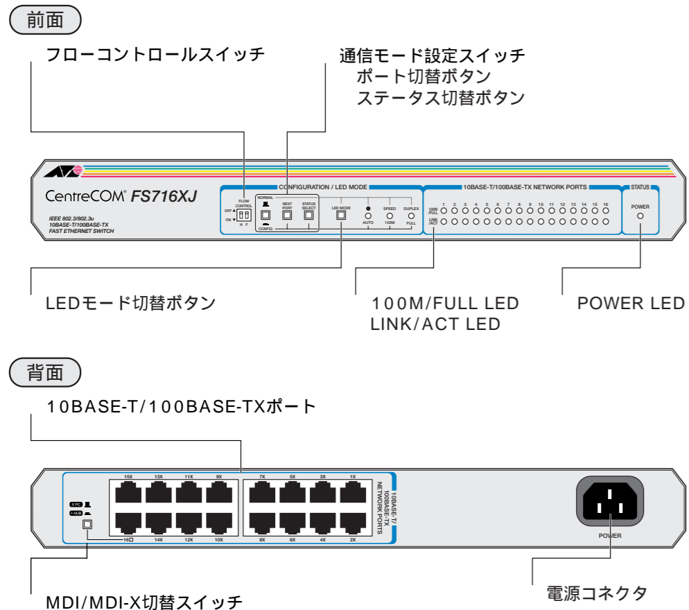
図1 外観図
