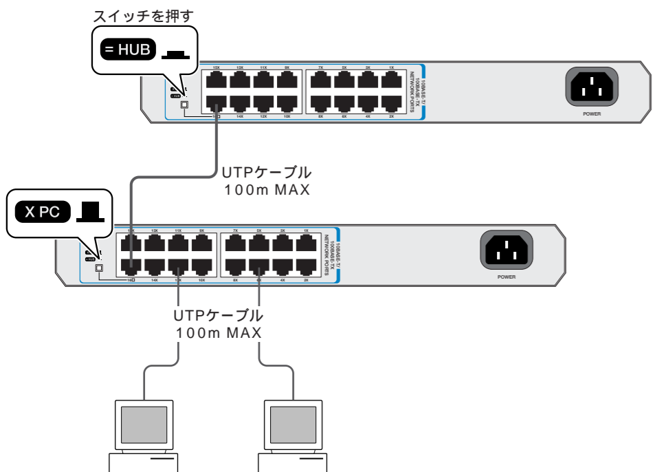
図5 カスケード接続の例
