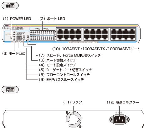
図 1 外観図
