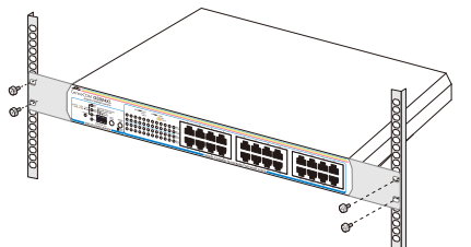
図 4 19 インチラックへの取り付け
