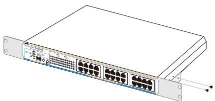
図 3 ブラケットの取り付け
