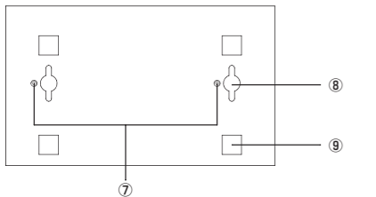
図 3 外観図 (底面、ポート下向き)
