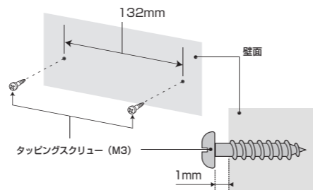
図 6 タッピングスクリューの間隔
