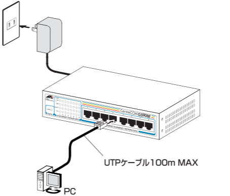
図 8 本製品への UTP ケーブルの接続
