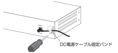
図 10 DC 電源ケーブルの固定
