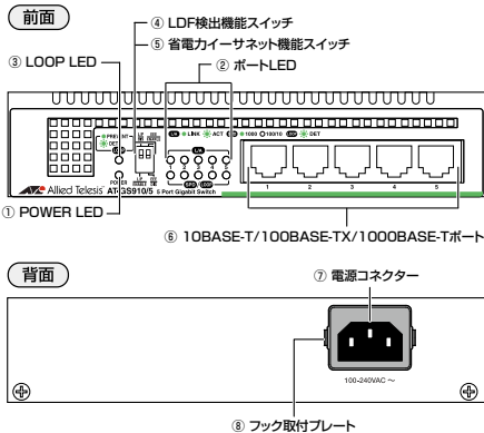
図 1 外観図
