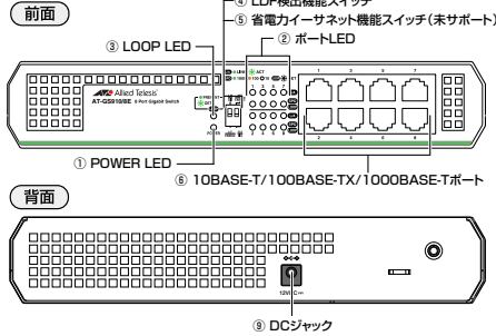
図 1 外観図
