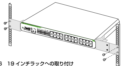
図 6 19 インチラックへの取り付け
