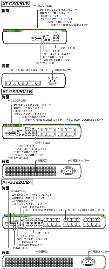
図1 外観図
