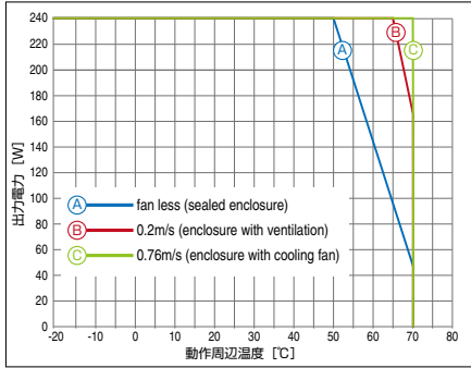
温度ディレーティングカーブ 230VAC
