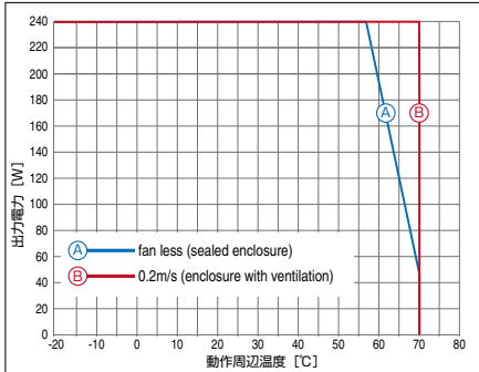
図 10 温度ディレーティングカーブ
