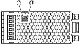
図2 天面外観
