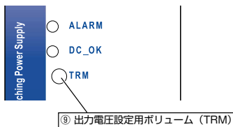
図4 前面外観：出力電圧設定用ボリューム
