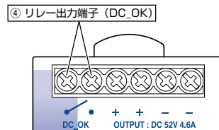
図6 前面外観：リレー出力端子
