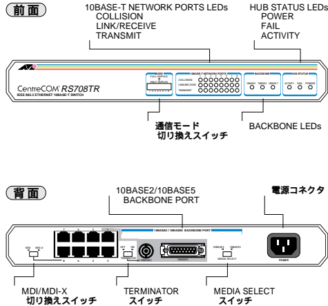
図1 外観図
