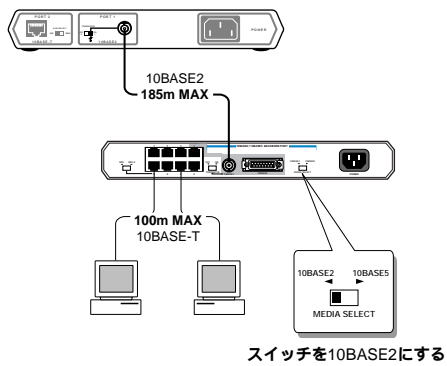
図2 10BASE2を接続した例
