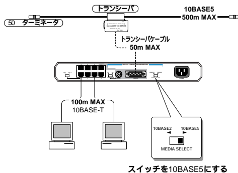
図3 10BASE5を接続した例
