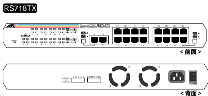
図1 外観図
