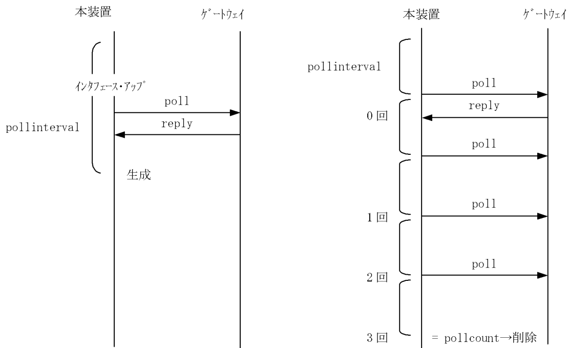
図 17-1 スタティック経路の動的監視による経路の生成、削除および再生成の例
