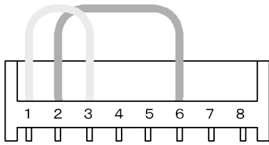
図 6-3 10BASE-T/100BASE-TX 用ループコネクタの概要図
