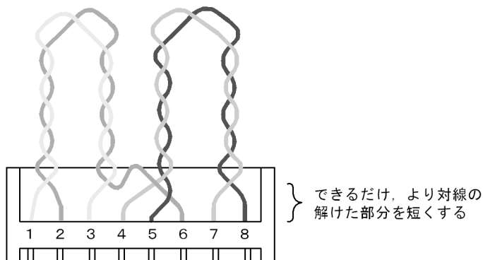
図 6-5 10BASE-T/100BASE-TX/1000BASE-T 用ループコネクタの概要図
