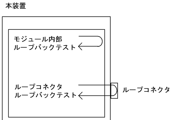
図 6-1 回線テスト種別ごとのフレームの折り返し位置
