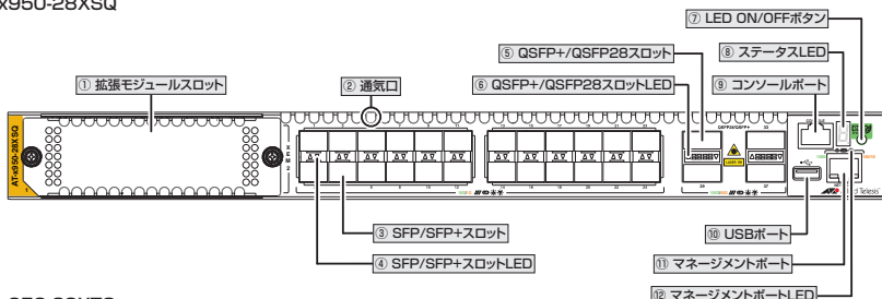
AT-x950-28XTQm
