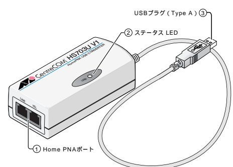
図1 外観図
