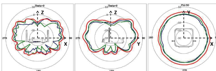
デュアルバンドアンテナ (5GHz)
