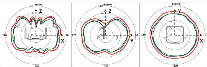
デュアルバンドアンテナ (2.4GHz)
