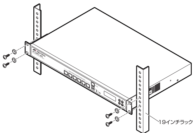
図 2.3.5 19 インチラックへの取り付け
