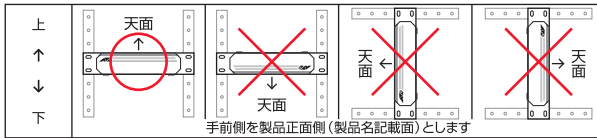
図 2.3.2 壁面への取り付け可能方向
