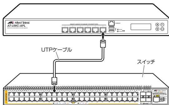
図 2.4.1 UTP ケーブルの接続
