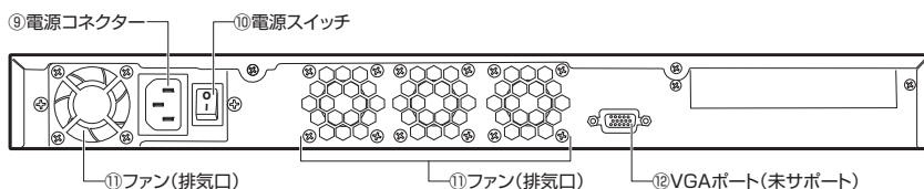
図 1.3.5 背面
