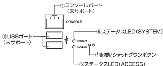
図 1.3.3 USB ポート周辺
