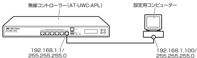
図 2.6.1 設定用コンピューターの接続
