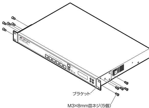
図 2.3.4 ブラケットの取り付け
