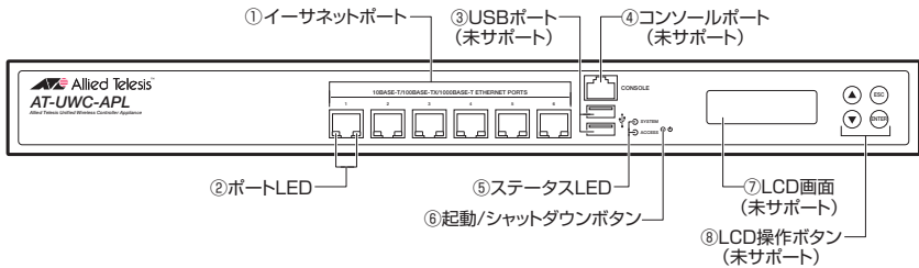
図 1.3.1 前面
