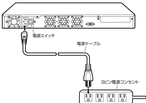
図 2.5.1 電源ケーブルの接続
