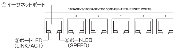
図 1.3.2 イーサネットポート
