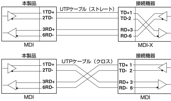
図 A.2.2 10BASE-T/100BASE-TX ケーブル結線図 (続)
