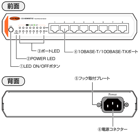
図1 外観図
