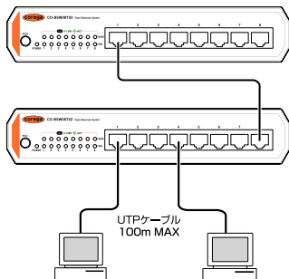
図9 カスケード接続 (図は CO-BSW08TX2)
