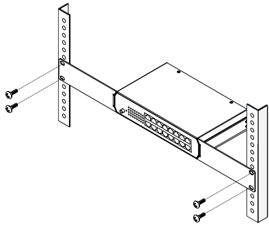
図4 19 インチラックへの取り付け (CO-BSW16TX2)
