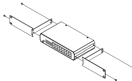
図 3 ブラケットの取り付け (CO-BSW16TX2)
