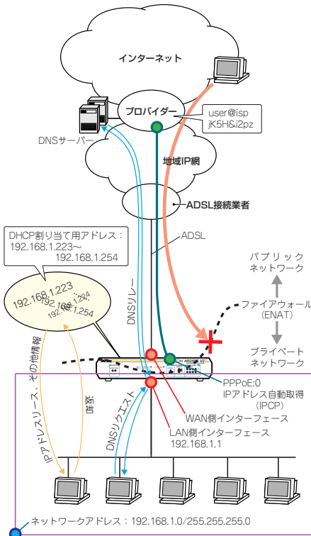
図 5.0.1 PPPoE による接続の模式図
