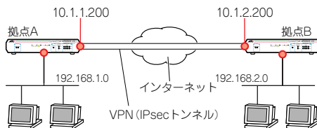
図 6.0.1 固定 IP アドレス同士の VPN 接続
