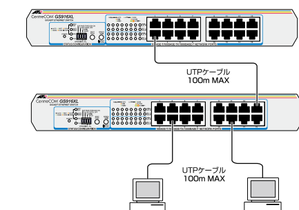
図6 カスケード接続
