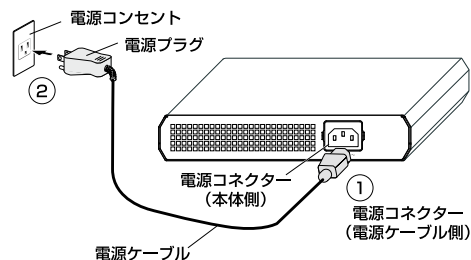
図 5 電源ケーブルの接続 (図は AT-GS910/8)
