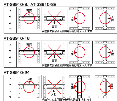
図 2 19 インチラック-mount キットを使用する場合の設置方向
