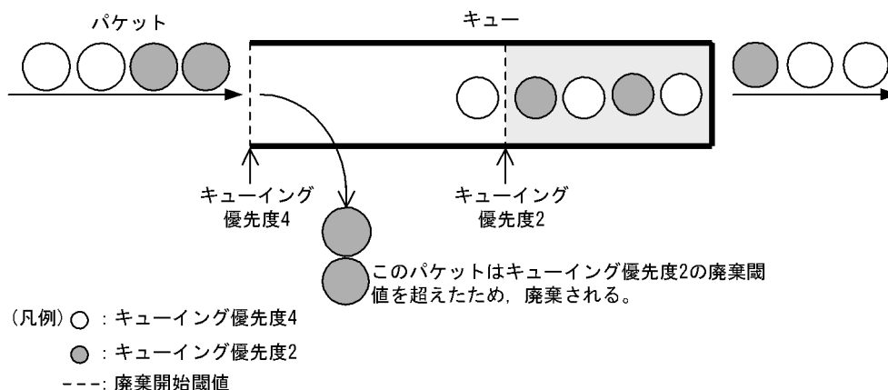
図 1-16 テールドロップの概念
