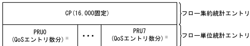
図 8-17 フロー統計エントリの実装位置
