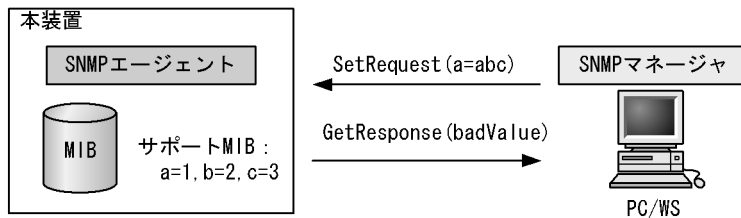
図 7-17 設定値のタイプが正しくない場合の SetRequest オペレーション例
