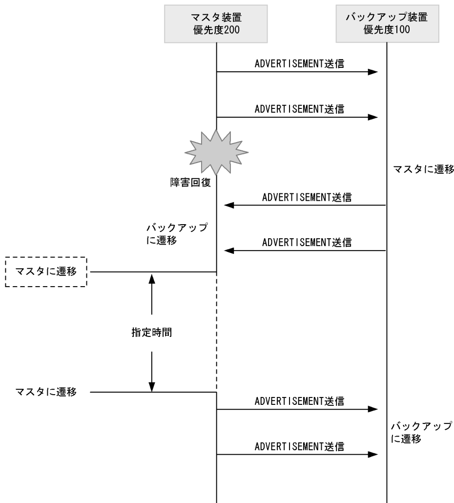
図 4-14 抑止タイマによるマスタ状態遷移
