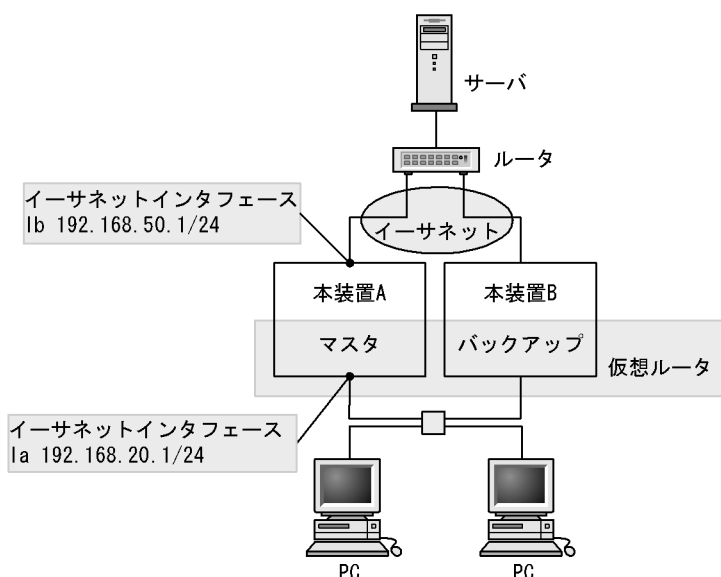
図 4-3 障害監視インタフェース
