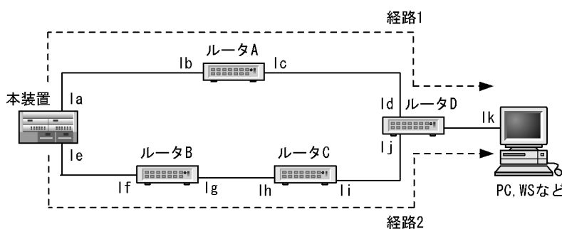
図 12-8 traceroute コマンドの使用例
