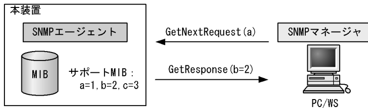
図 7-9 GetNextRequest オペレーション
