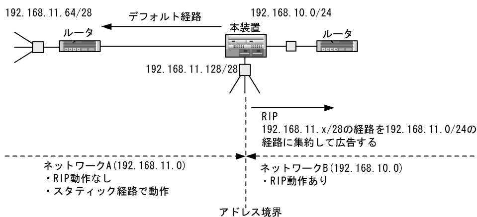
図 13-3 noinstall サブコマンドが必要な構成例
