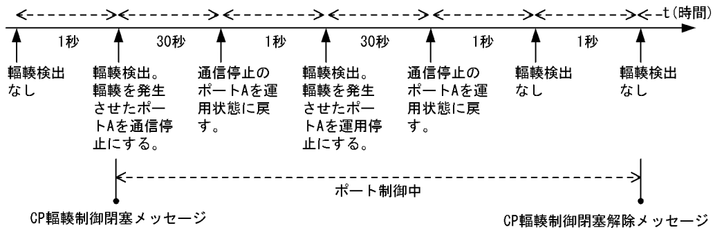
図 5-2 CP 輻輳制御メッセージ出カタイミングの例 (CP 輻輳制御時間が 30 秒の場合)
