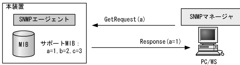
図 7-8 GetRequest オペレーション (SNMPv3)
