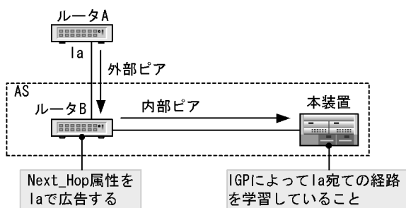
図 13-2 Next_Hop 解決
