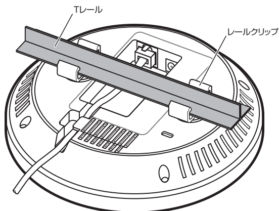
図 2.3.9 T レールへの取り付け
