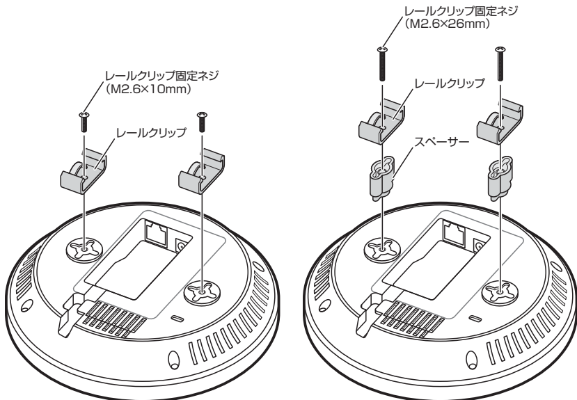
図 2.3.8 レールクリップの取り付け
