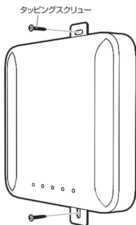
図 2.3.7 設置面への取り付け
